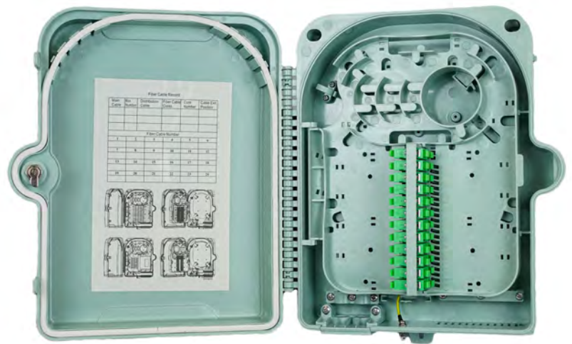
PN: HE-48NID-01
